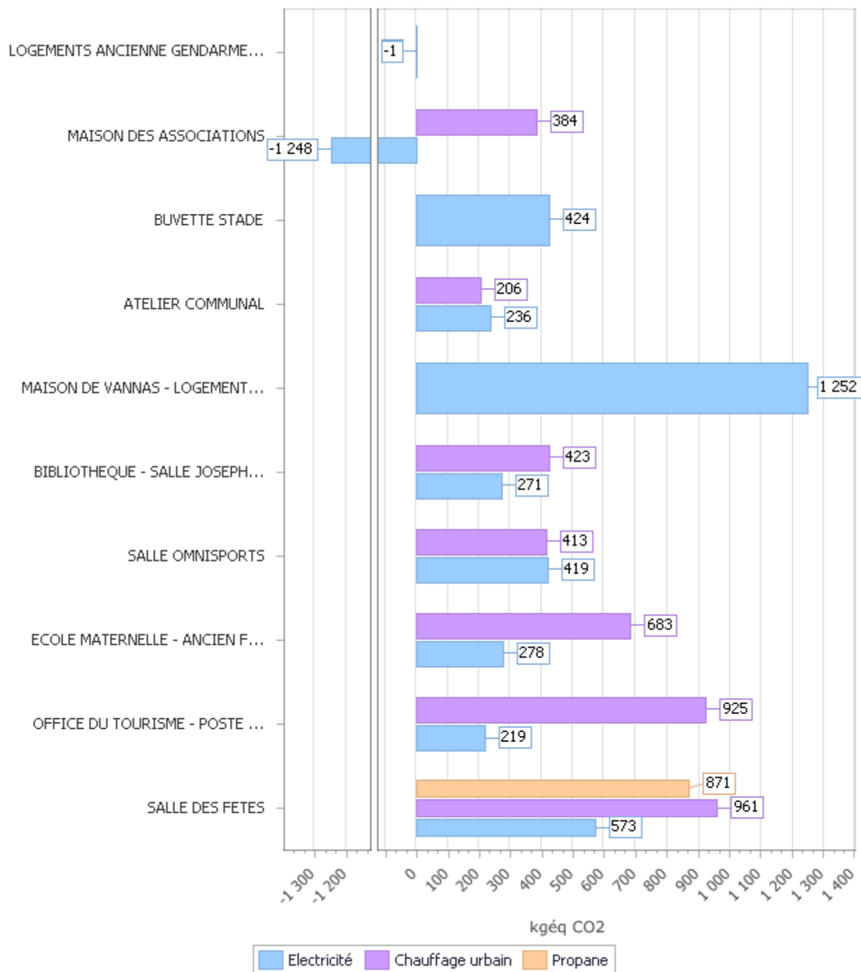
Figure 22 : Emissions de GES par énergie et par établissement (2015) (Top 1 à 10)
