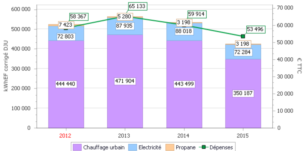
Figure 1 : Evolution des consommations corrigé DJU et dépenses du patrimoine bâti
