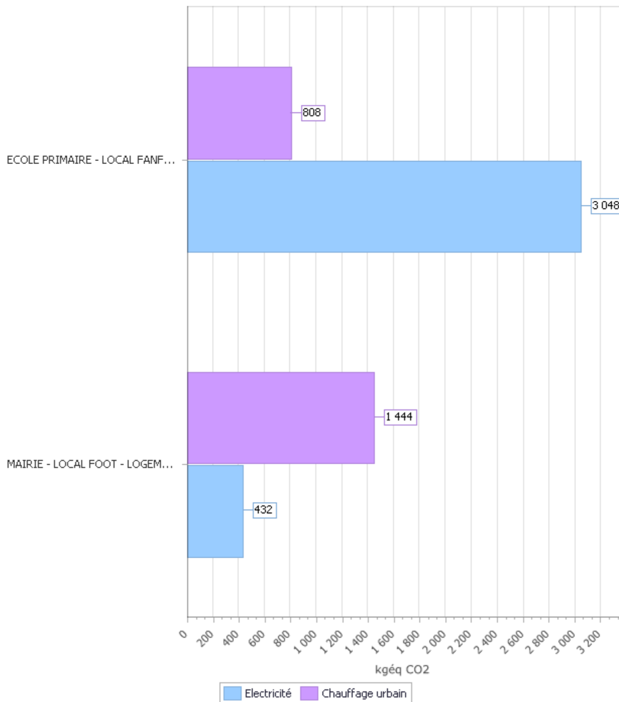
Figure 23 : Emissions de GES par énergie et par établissement (2015) (Top 11 à 12)
