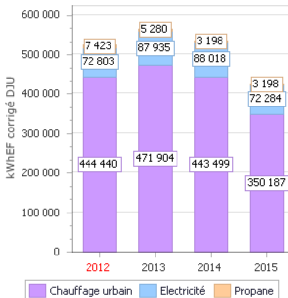
Figure 4 : Evolution des consommations corrigé DJU par énergie
