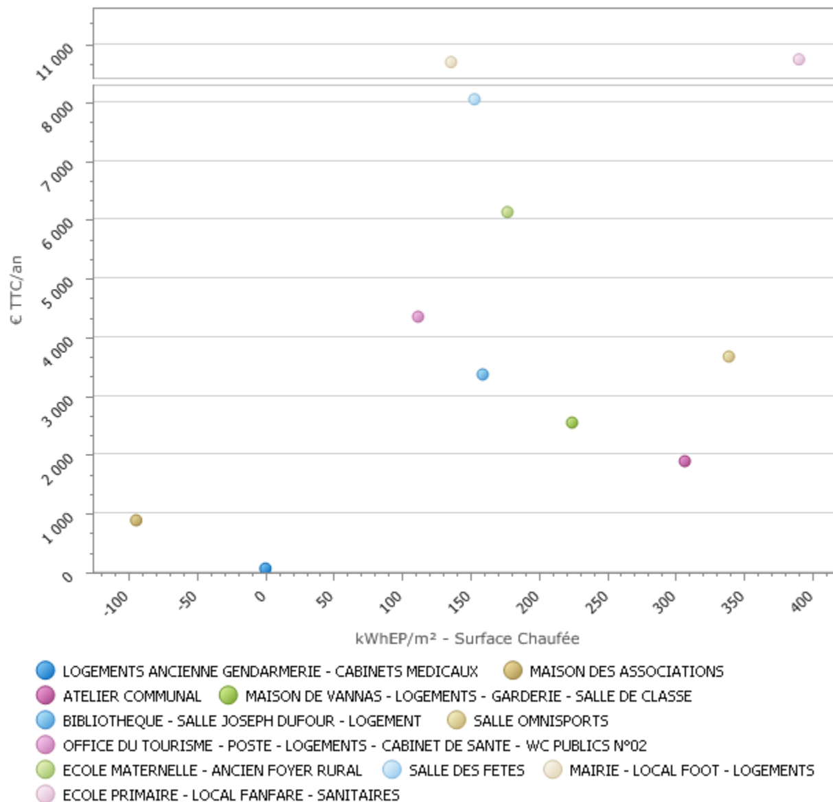
Figure 26 : Classement des établissements par performance énergétique et dépenses (2015)
