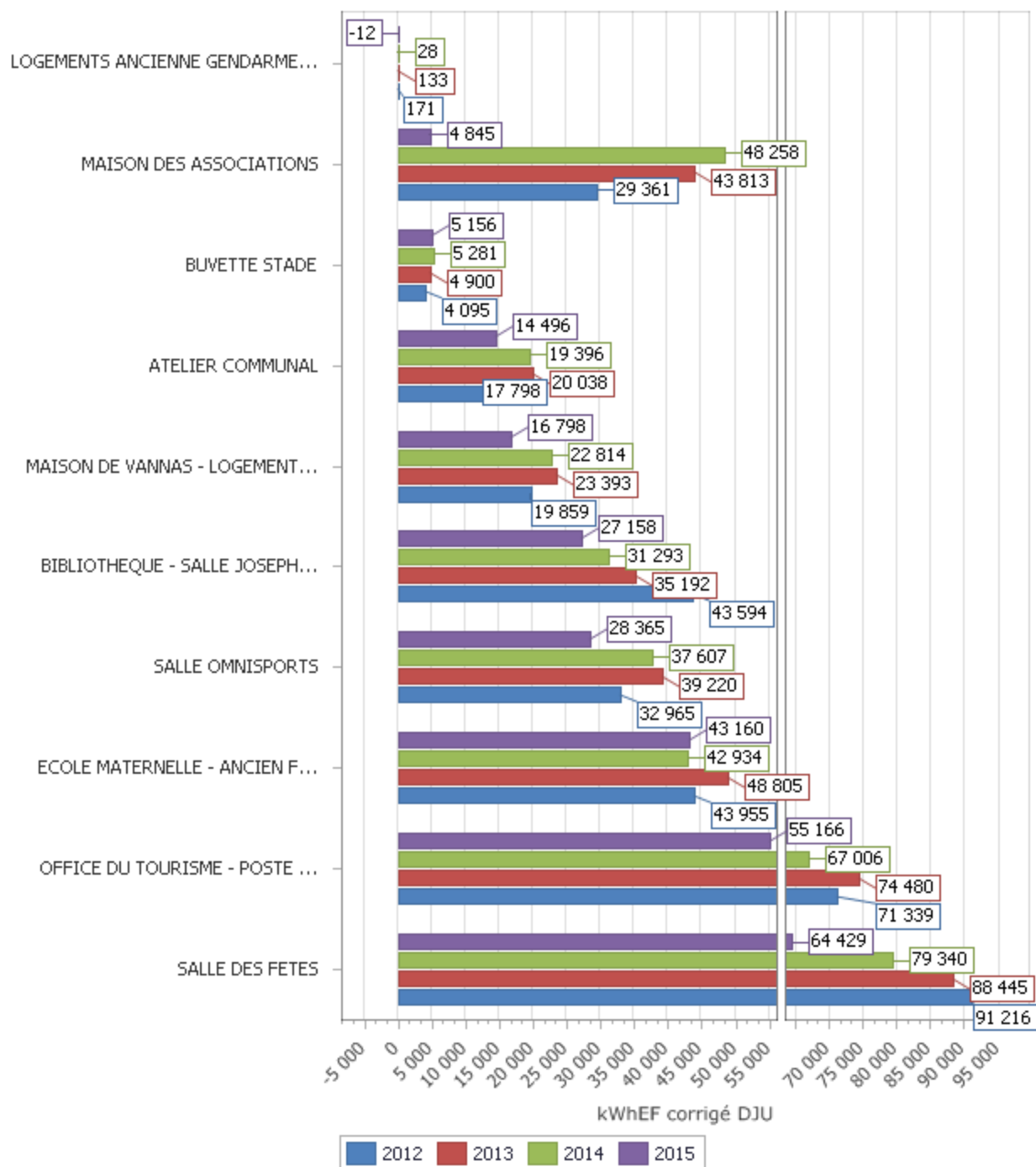
Figure 9 : Evolution des consommations corrigé DJU par établissement (Top 1 à 10)
