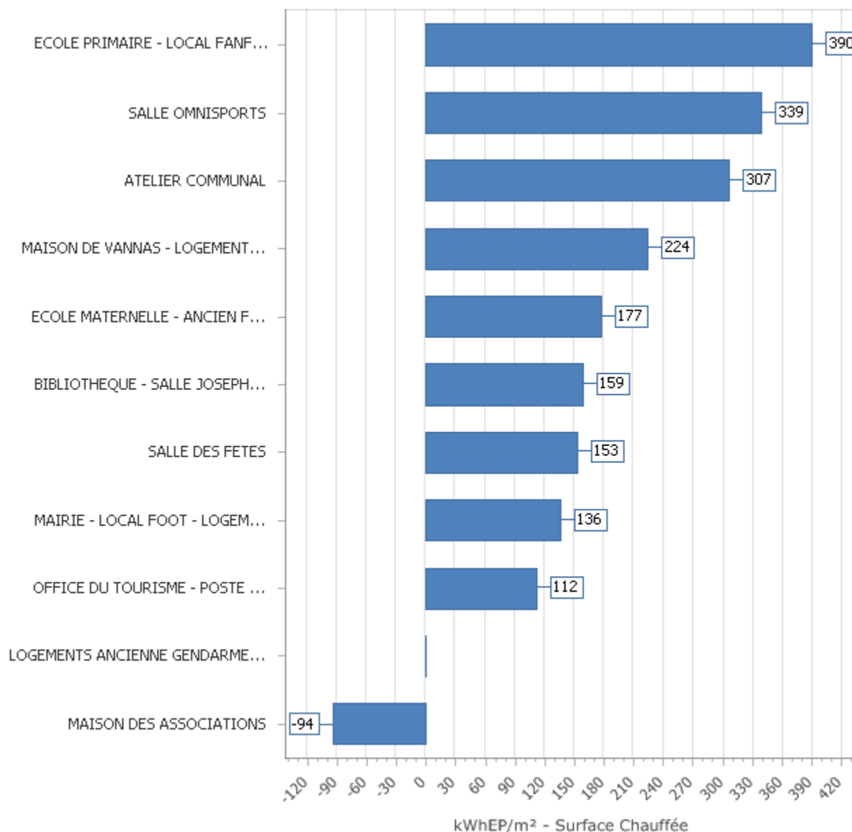
Figure 24 : Classement des établissements suivant la performance énergétique (2015)
